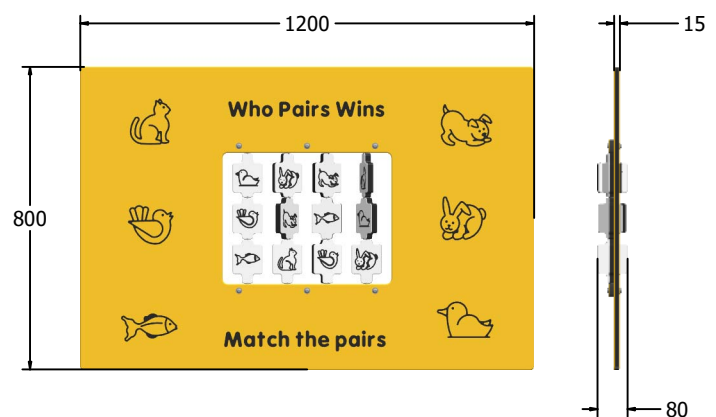
FIWPWINS3 FIWPWINS3-AL-WP
