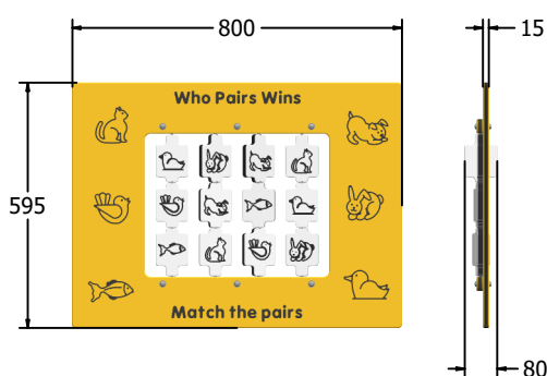
FIWPWINS6 FIWPWINS6-AL-WP
