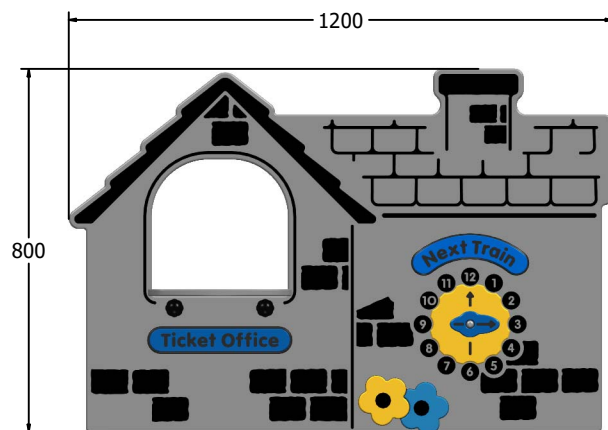
FITICK3
